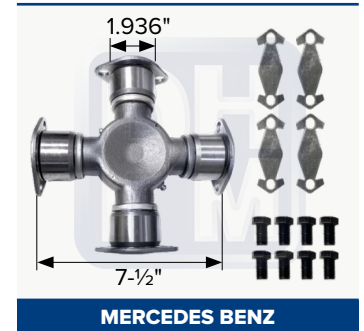
Cruceta de dirección
