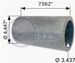
MACK OEM 10QK149 Buje para muelle tipo Mack
