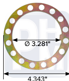
MERITOR OEM Rondana de eje
