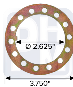
MERITOR OEM 1229G1021 Rondana de eje
