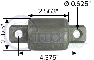
KENWORTH OEM C136001 Buje de torsión de alto confinamiento
