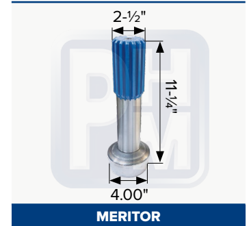
OEM 6-40-521
