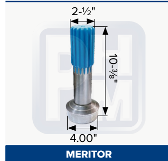
OEM 6-40-541
