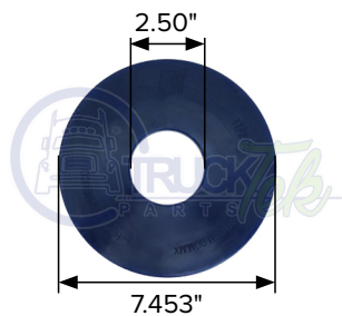
MERITOR OEM 21226663 Rondana de desgaste para meritor
