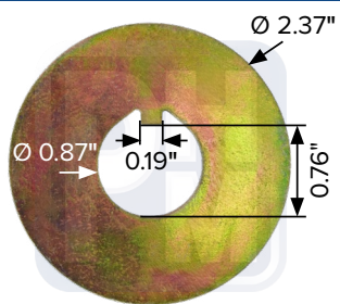
OEM Rondana de mango delantero
