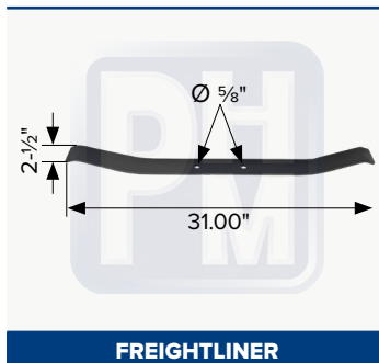
Soporte muelle de transmisión
