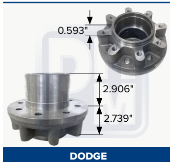
Maza trasera D-350 frenado de disco
