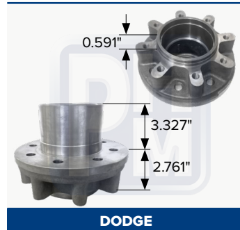
Maza trasera DODGE RAM 4000 de 8 birlos
