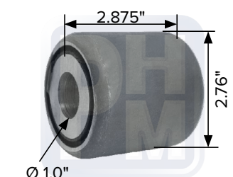
NEWAY OEM 90008264 Buje para barra angular de 2-3/4" X 1"
