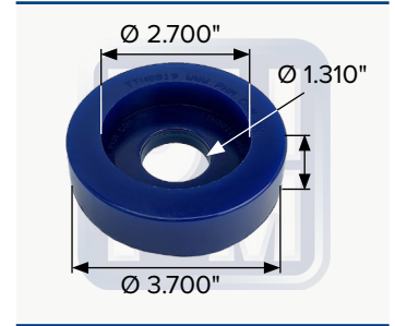
OEM 6802410218, J197911 Complemento de soporte para motor superior trasero
