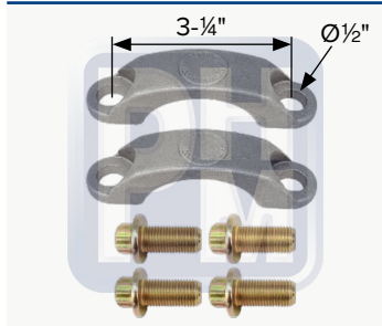
OEM 2500674C91, 3947699 Juego de abrazaderas para cruceta
