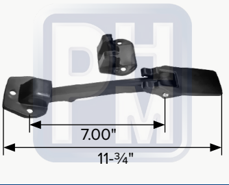
Gancho para cofre
