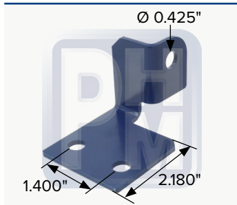
INTERNATIONAL OEM 3565269C1 Soporte para cable de seguridad
