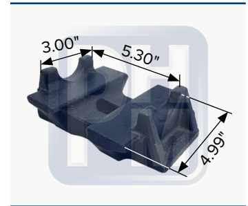
Asiento de muelle a 6° tipo International
