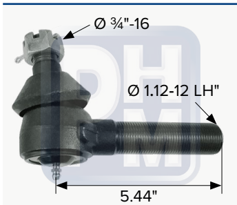
Terminal International Navistar Autobus Escolar
