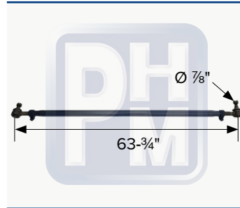
OEM 3818387C91 Brazo de Dirección International 4700
