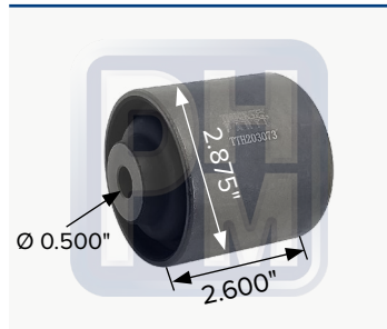
OEM 3574680C1 Buje para soporte de cabina
