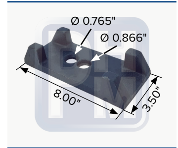
OEM 493480C2 Asiento de muelle
