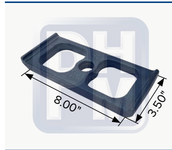
OEM 493721C3 Espaciador de muelle "Z" 3½"
