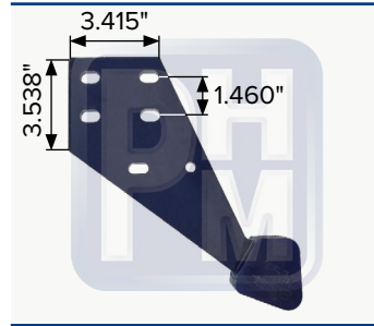
OEM 3548892C3 Guía de cofre para International
